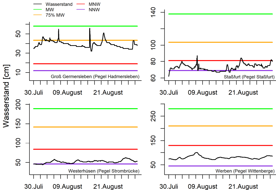
Abbildung 1: Wasserstände an Pegeln in der Nähe der Sondenstandorte. Wasserstand = niedrigster jemals gemessener Wasserstand (NNW, violett) ; Wasserstand = mittleres Niedrigwasser (MNW, rot) ; Wasserstand = 75% Mittelwasser (75% MW, orange) ; Wasserstand = Mittelwasser (MW) .
